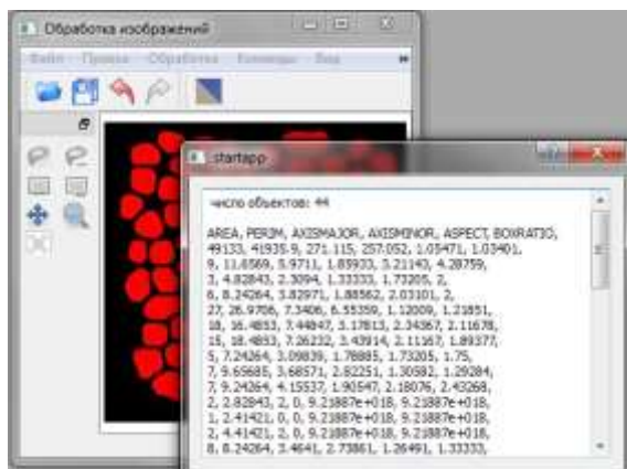
Рисунок 10 Копия экрана программы ТІР для анализа наоперехности
