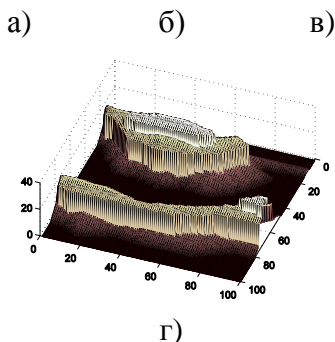
Рисунок 4 – Исходное полутоновое изображение (а), полутоновое изображение, умноженное на 256 (б), псевдо-дистанционная карта (в), и 3D-представление псевдо-дистанционной карты (г)
